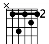
D7
