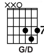
G/D
