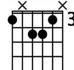
Gmaj7
