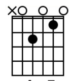
Am7v
