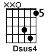
Dsus4
